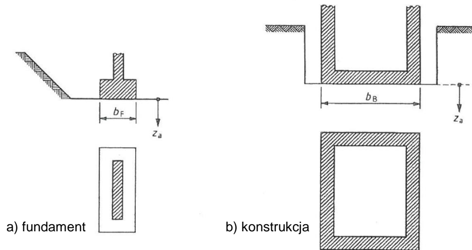
Rys. 4-5 Proponowana głębokość rozpoznania podłoża budowli o dużej wysokości i konstrukcji inżynierskich z zgodnie z [74]
