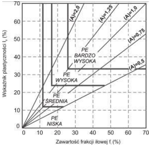
Rys. Z. 9-1 Nomogram do oceny potencjalnej ekspansywności (PE) gruntów aktywność - A = I_p/f_i [9]
