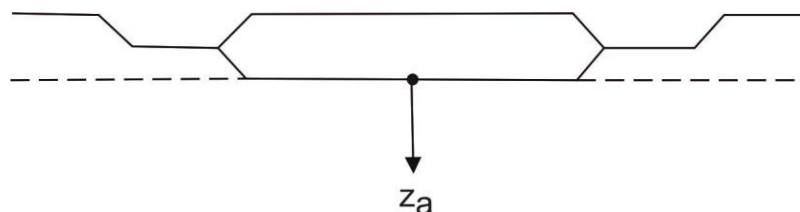
Rys. 4-2 Proponowana głębokość rozpoznania podłoża obiektów liniowych zgodnie z [74]
