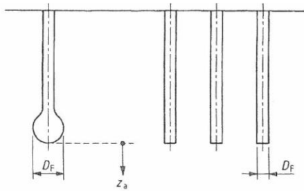
Rys. 4-7 Proponowana głębokość rozpoznania podłoża budowli o dużej wysokości i konstrukcji inżynierskich z zgodnie z [74]
