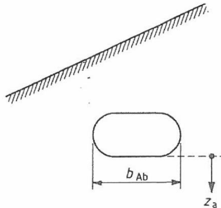
Rys. 4-6 Proponowana głębokość rozpoznania podłoża małych tuneli i komór podziemnych (np. przejść pod torami) z zgodnie z [74]
