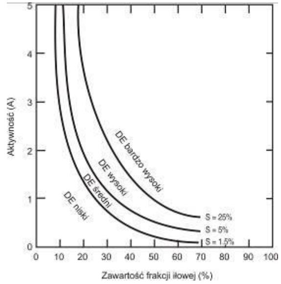
Rys. Z. 9-2 Wykres klasyfikacji stopni ekspansji (DE) oraz potencjał pęcznienia (S) aktywność - A = I_p/(f_i-5) [9]
